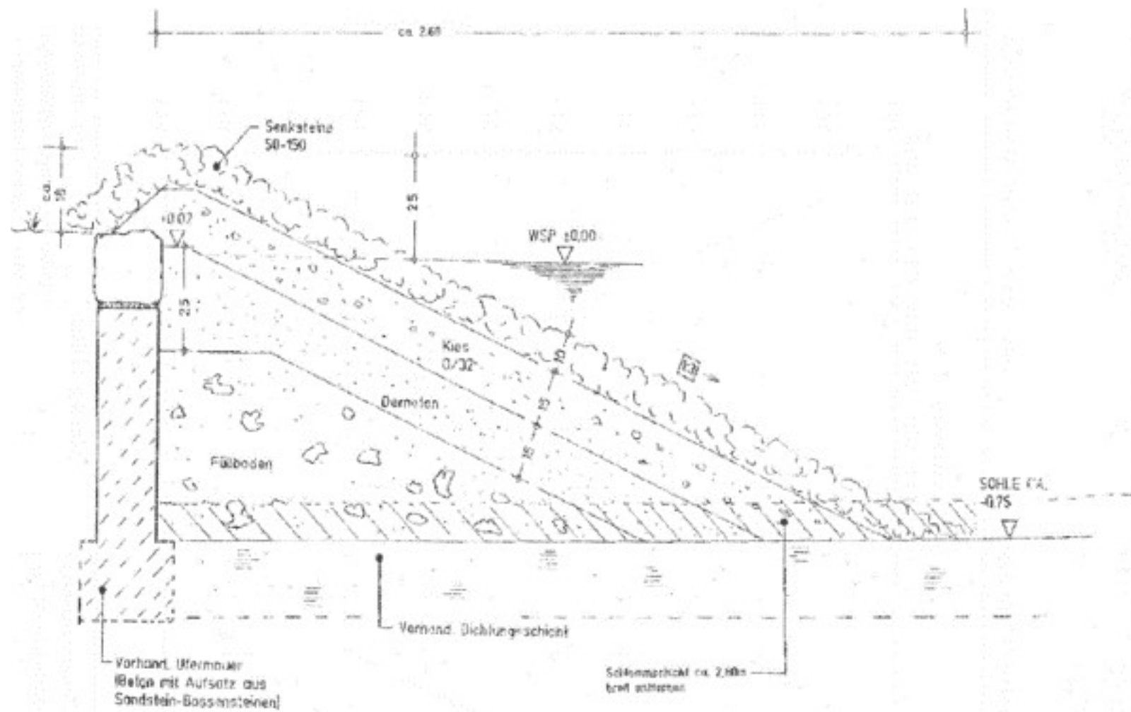
QUERSCHNITT A-A', 1:10
